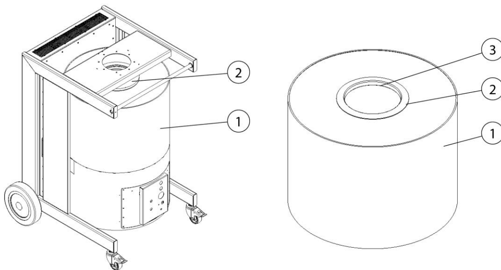
Abb. 2: Montage
