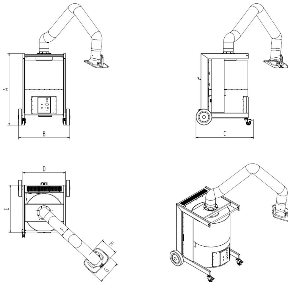
Abb. 15: Maßblatt
