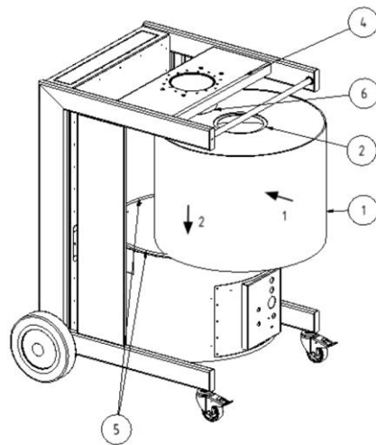
Abb. 6: Filterwechsel
