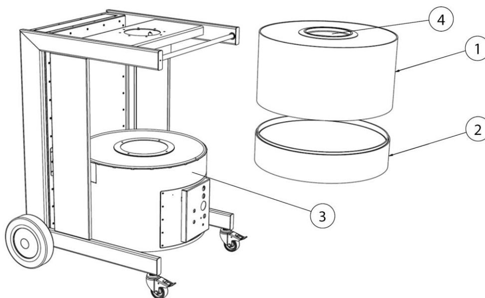
Abb. 8: Filterwechsel
