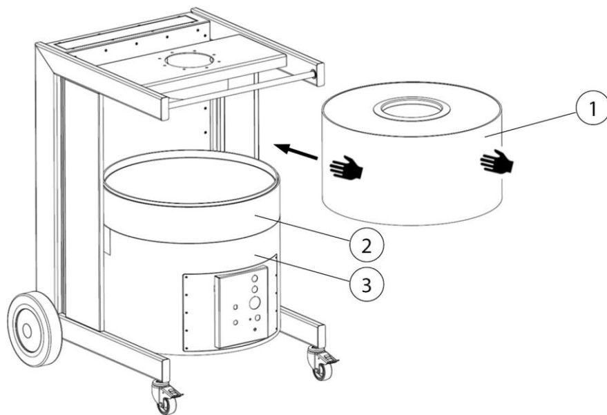
Abb. 12: Filterwechsel – Filterelement einsetzen
