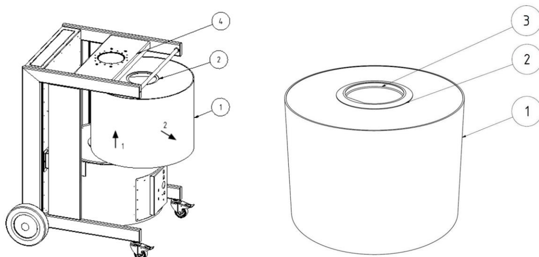
Abb. 5: Filterwechsel
